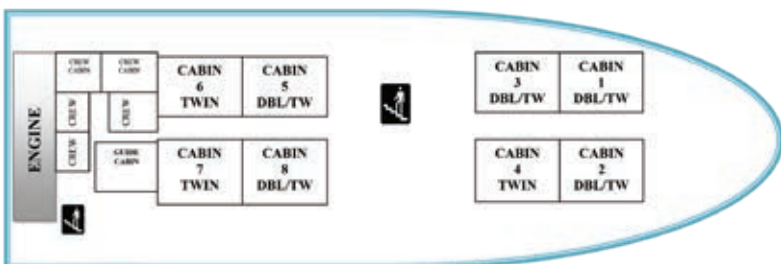
Cubierta Inferior
